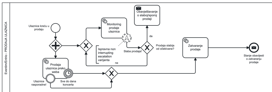
Slika 26. Primjer modeliranog procesa ORGANIZACIJA KONCERTA U PULSKOJ ARENI s korištenim non-interrupting escalation boundary eventom vezanim za aktivnost "Monitoring prodaje ulaznica" kojim se hvata eskalacija "Evidentirana slaba prodaja ulaznica" i pokreće se slijed aktivnosti marketinškog tima za poboljšanje prodaje ulaznica, dok se glavna aktivnost normalno nastavlja izvoditi.
